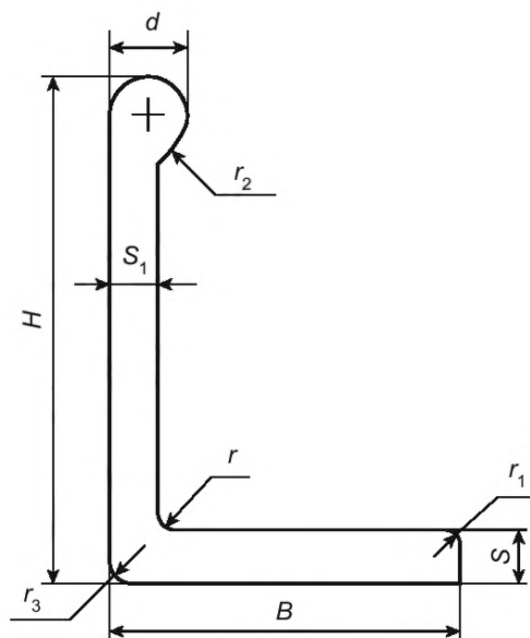
Рисунок 1 — Прессованный бульбообразный профиль уголкового сечения
