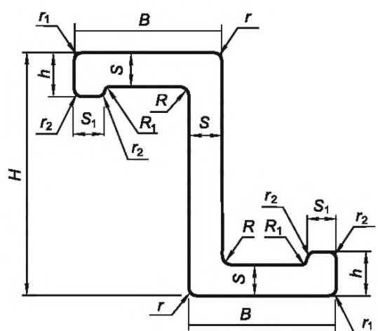
B — длина; H — высота; S, S_1 — толщина; r, r_1, r_2 — радиусы притупления; R, R_1 — радиусы скругления Рисунок 1 — Прессованный прямоугольный профиль фасонного зетового сечения
