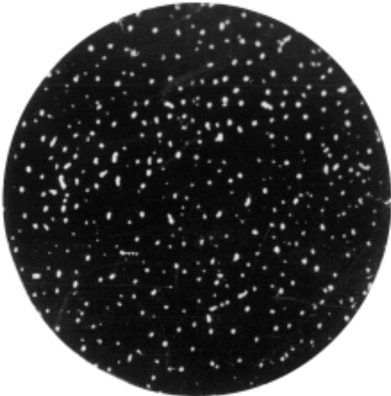
Шкала для оценки цементитной сетки в инструментальной нелегированной стали (500 \times )
