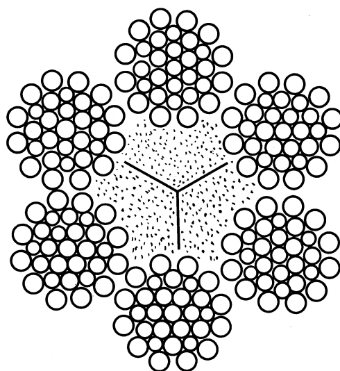
Шестипрядный канат 6×31+1 о. с.; 6×31=186 проволок с органическим сердечником (прядь каната 1+6+6/6+12).
