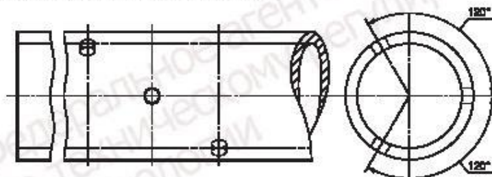
Рисунок Г.1 — Эталонный образец с тремя отверстиями
