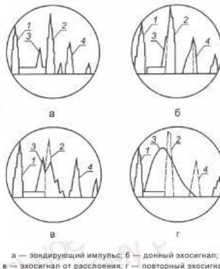
Рисунок В.1 — Вид эхосигналов на экране дефектоскопа
