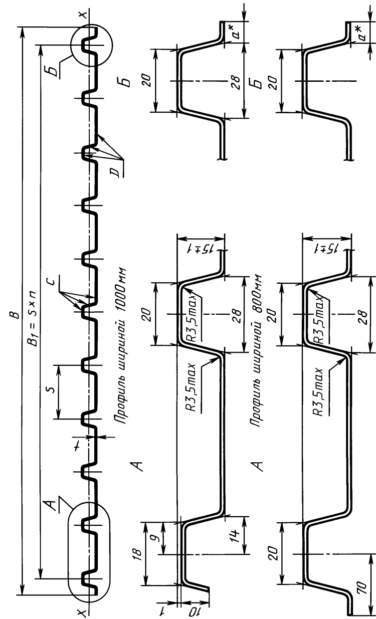
Рисунок 8 — Профилированный лист типа С высотой 15 мм
