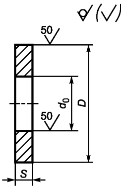
Рисунок 16 — Шайба (поз. 17 на рисунке 1)
