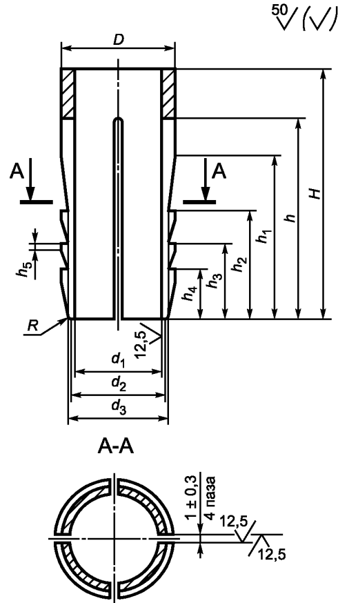
Рисунок 14 — Разжимная цанга (поз. 15 на рисунке 1)
