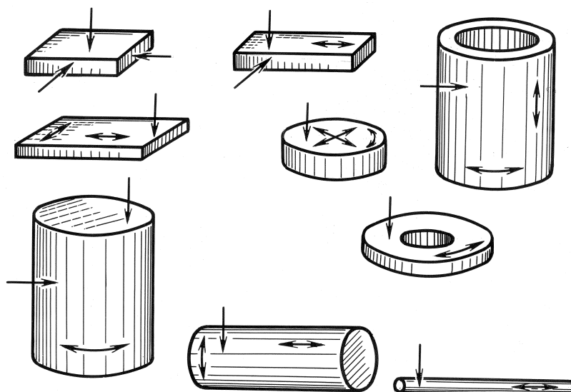
Примеры прозвучивания поковок простой формы
