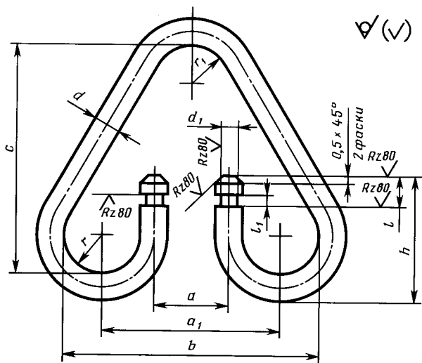
Размеры в миллиметрах
