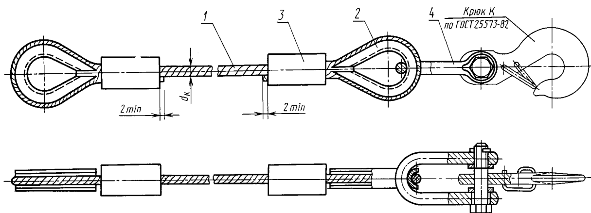
Канатная ветвь с переходным звеном
