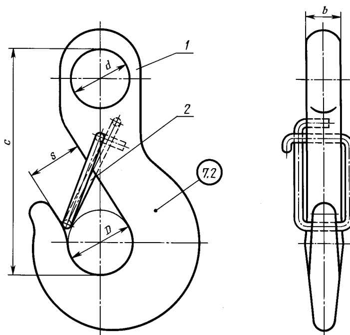
1 — крюк; 2 — замок
