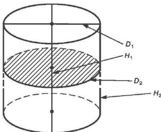
Рисунок Ж.1 — Схема измерения геометрических размеров брикета
