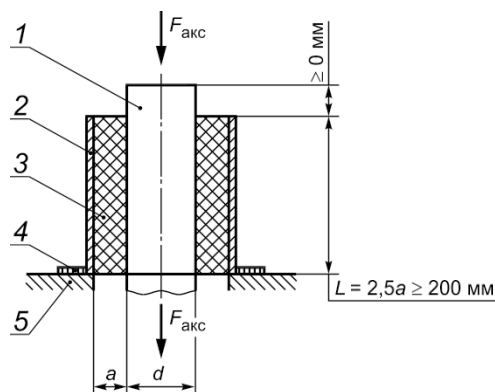
1 — стальная труба; 2 — защитная оболочка; 3 — ППУ изоляция; 4 — направляющее кольцо; 5 — плита основания машины для испытания; a — толщина изоляции; F_{\text{акс}} — прилагаемая нагрузка (внизу — альтернативный способ приложения нагрузки); d — см. экспликацию к формуле (4)
