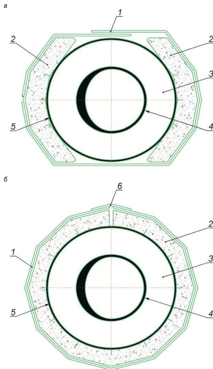
1 — оболочка из синтетического материала; 2 — компенсационный мат; 3 — ППУ изоляция; 4 — стальная труба; 5 — ПЭ оболочка; 6 — фиксирующая клейкая лента
