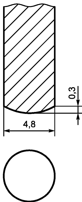
a — Скругленный наконечник
