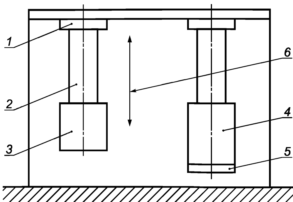
1 — испытательный стенд; 2 — nippleный конец трубы; 3 — nippleная предохранительная деталь; 4 — муфта; 5 — муфтовая предохранительная деталь; 6 — направление движения
