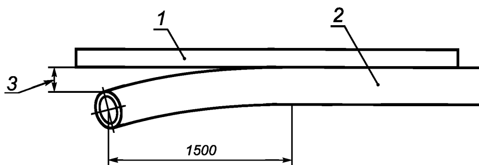
Рисунок D.14 — Измерения концевой прямолинейности
