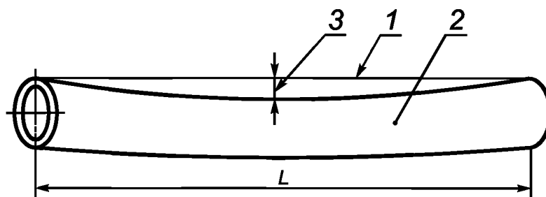
Рисунок D.13 — Измерения прямолинейности по всей длине
