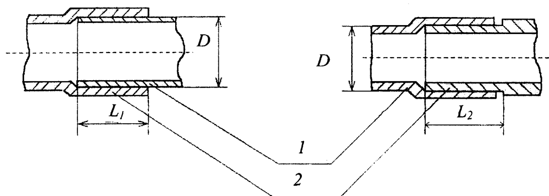
1 – труба; 2 – фитинг; D – диаметр соединяемых труб; L_1 – длина внутреннего участка под пайку для фитинга, охватывающего трубу в соединении; L_2 – длина наружного участка под пайку для фитинга, охватываемого трубой в соединении.
