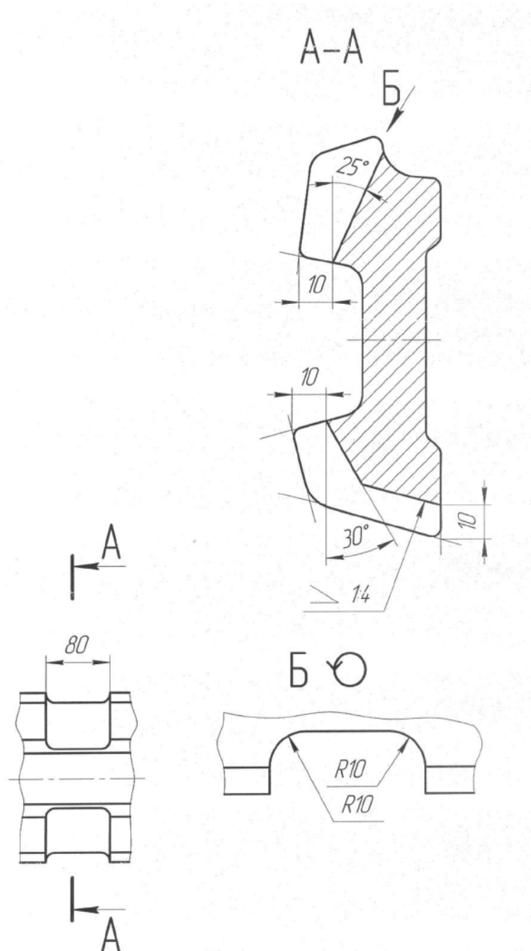
Рисунок 5 – Размеры поперечной фрезерованной канавки в накладках исполнений 3 и 5 для алюминотермитной сварки
