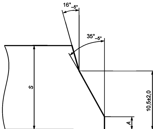
A — ширина торцевого притупления, S — толщина стенки
