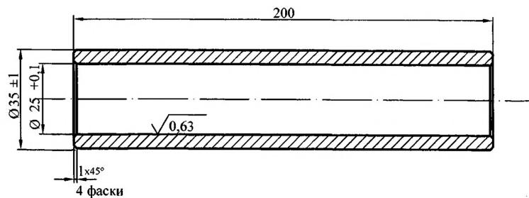
Рисунок А1 — Калибр для проверки кривизны шурупов
