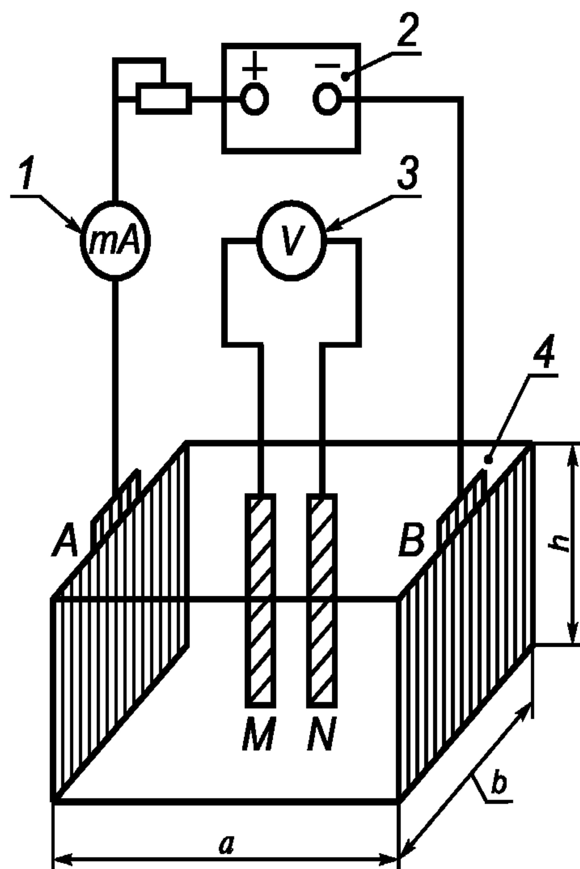
1 — миллиамперметр; 2 — источник тока; 3 — вольтметр; 4 — измерительная ячейка размерами a , b ; h (см. А.2.2); A и B — внешние электроды; M и N — внутренние электроды
