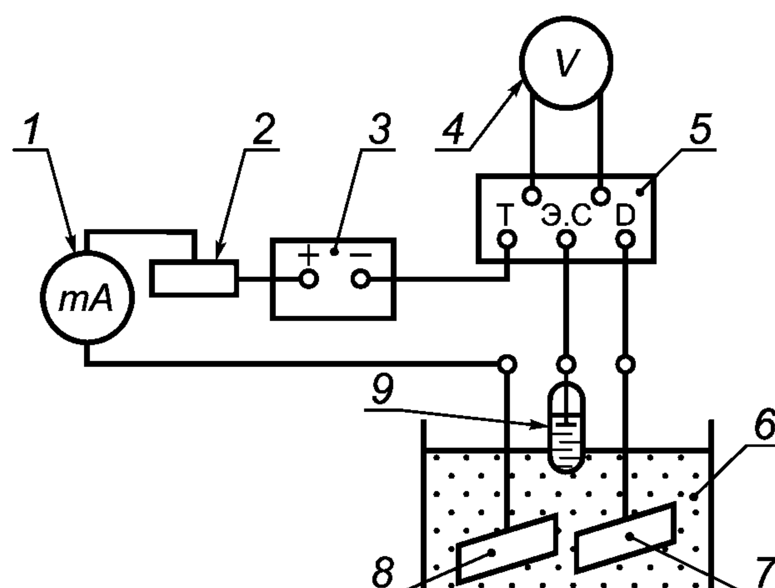
1 — миллиамперметр; 2 — регулируемое сопротивление; 3 — источник постоянного тока; 4 — вольтметр; 5 — прерыватель тока с клеммами для подключения электродов: Т — вспомогательного, Э.С — сравнения, D — рабочего; 6 — ячейка; 7 — рабочий электрод; 8 — вспомогательный электрод; 9 — электрод сравнения
