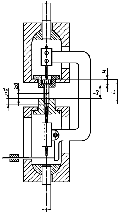
Рисунок 6 — Тензометр, установленный на болт в самоцентрирующих зажимах
