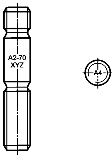
Рисунок 5 — Маркировка шпилек — альтернативные формы
