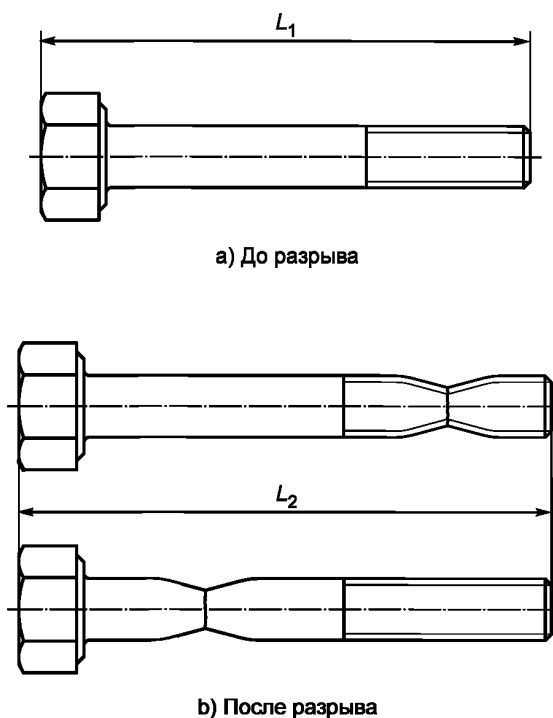
Рисунок 8 — Определение удлинения после разрыва A
