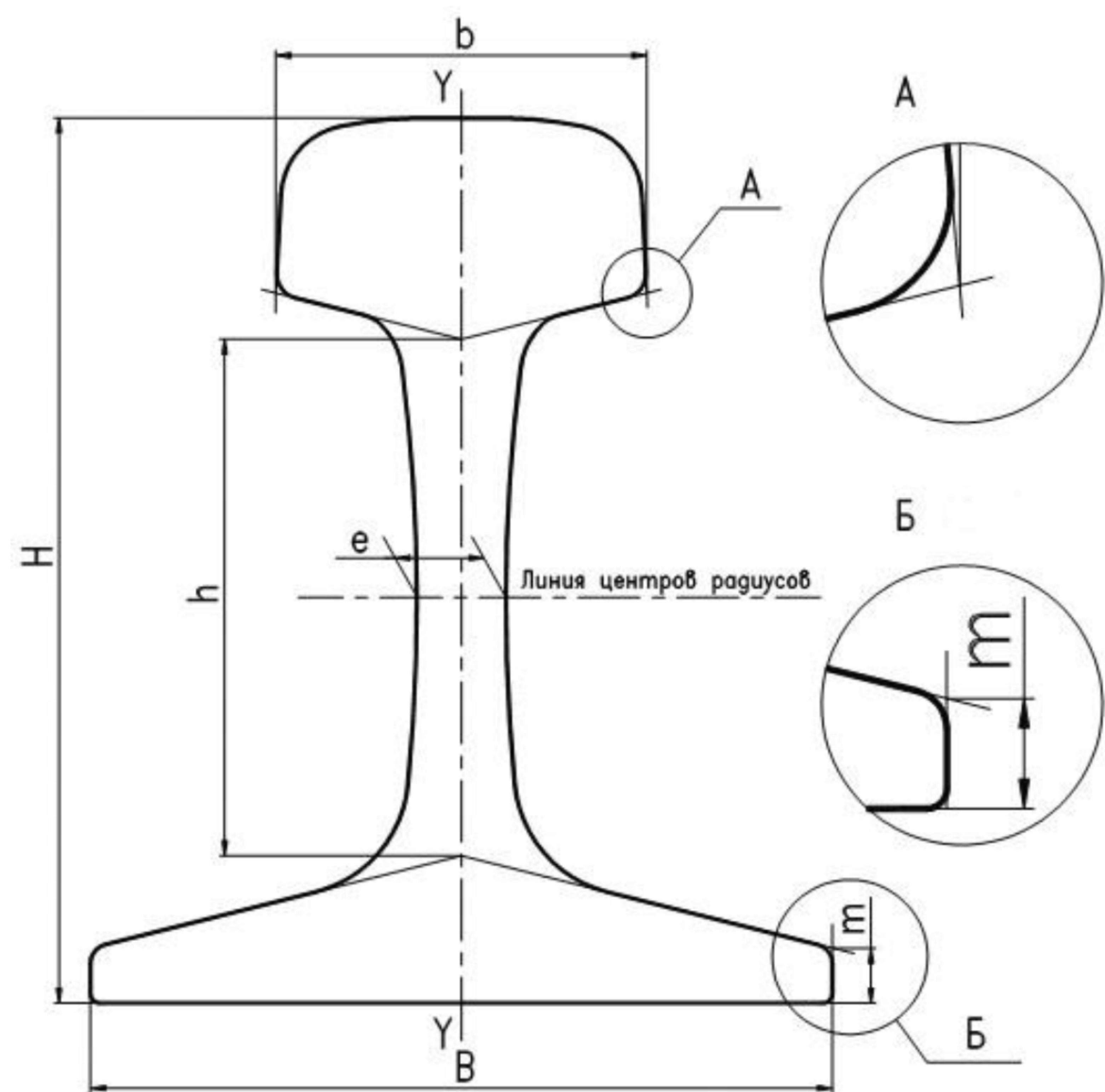
Рисунок 1 – Конструкция и основные размеры поперечного сечения рельсов
