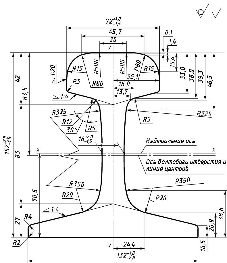
Рисунок 1 — Поперечное сечение рельса типа РП50
