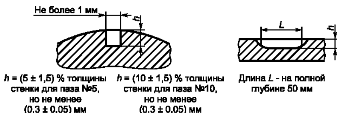
а - пазы типов №5 и №10
