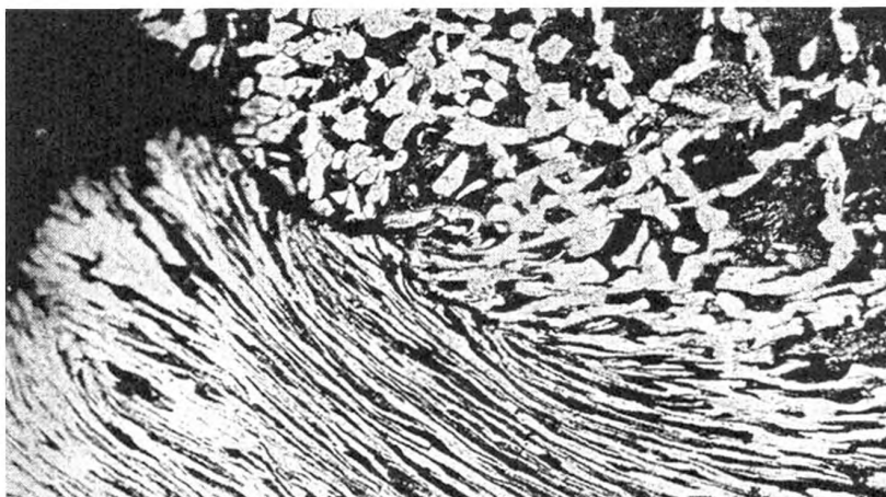
Рисунок А.1 — Микроструктура металла у намина (ув. 200×)
