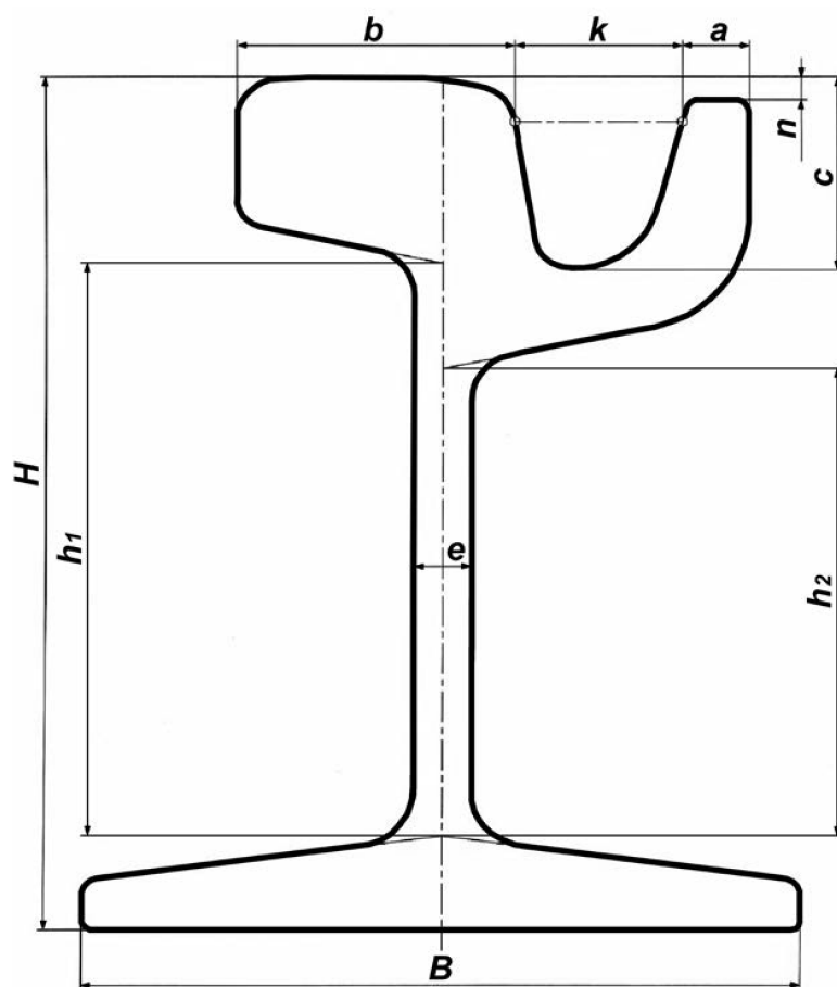
Рисунок 1 — Основные размеры поперечного сечения желобчатых рельсов
