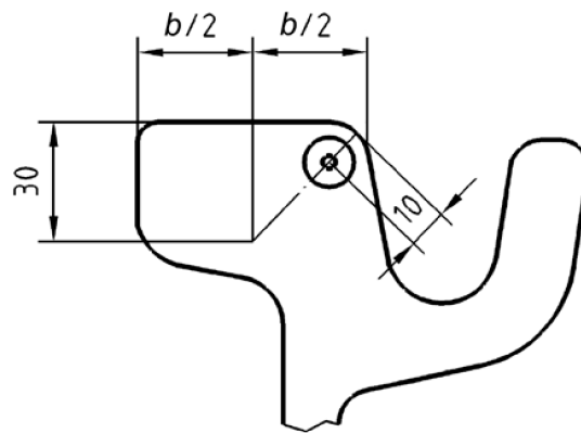
Рисунок 3 — Расположение образца для определения механических свойств
