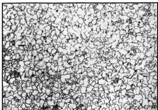
Балл 7, 100 \times , химическое травление
