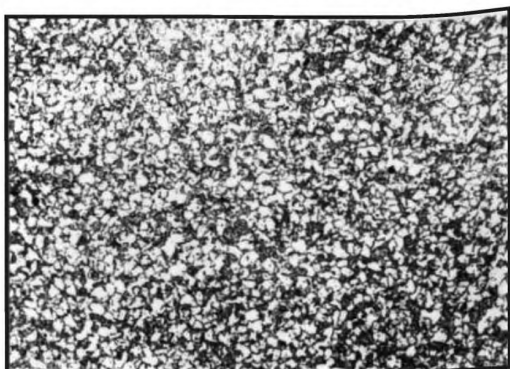
Балл 4, 100 х , электролитическое травление
