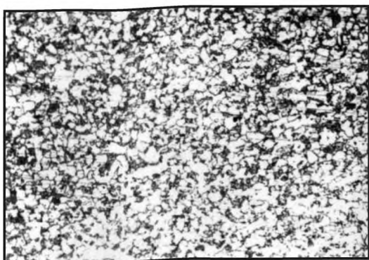
Балл 5, 100 \times , электролитическое травление
