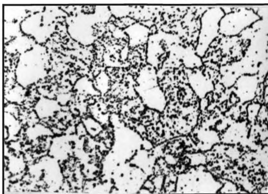
Балл 3, 500 х , электролитическое травление
