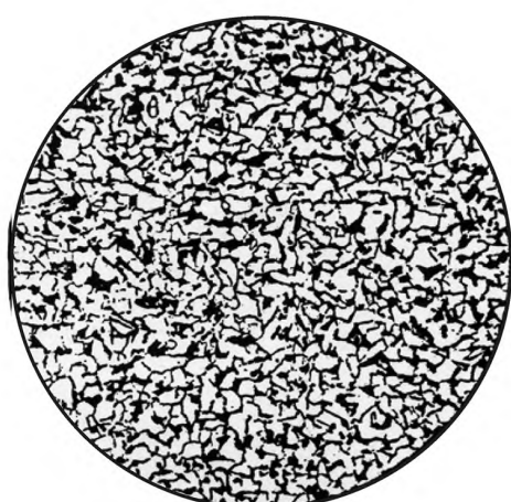
Балл 0
