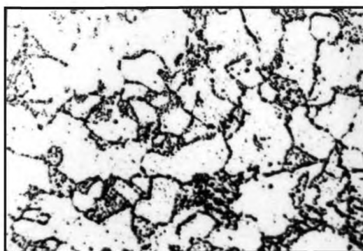
Балл 5, 500 \times , электролитическое травление
