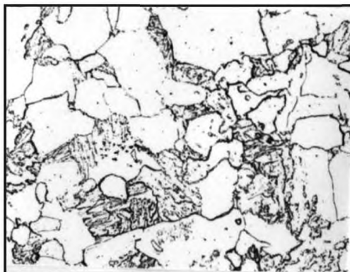
Балл 4, 500 х , химическое травление
