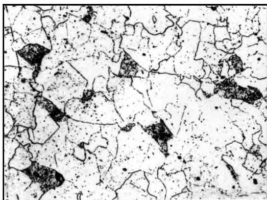
Балл 6, 100 х
