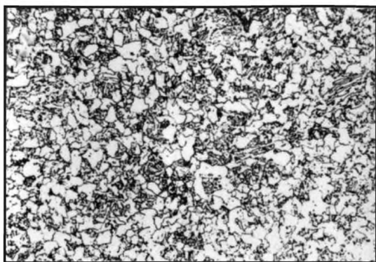
Балл 3, 100 х , химическое травление
