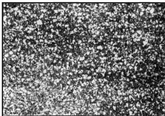
Балл 3, 100 х , электролитическое травление
