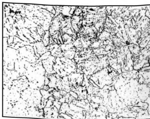
Балл 1, 500 \times , химическое травление
