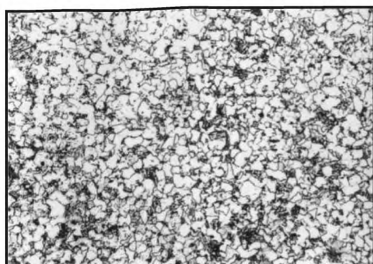
Балл 6, 100 \times , химическое травление
