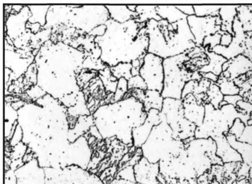
Балл 5, 500 х , химическое травление
