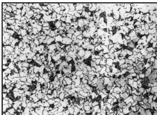
Балл 4, 100 x
