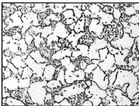
Балл 4, 500 х , электролитическое травление
