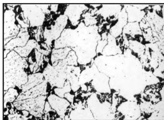
Балл 8, 500 х , электролитическое травление
