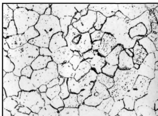
Балл 7, 500 \times , химическое травление
