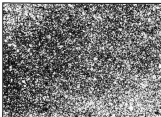
Балл 1, 100 \times , электролитическое травление
