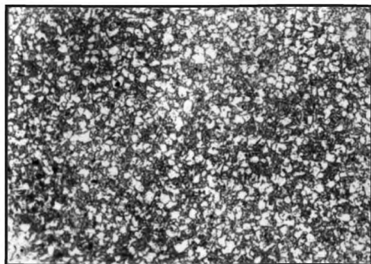
Балл 2, 100 х , электролитическое травление
