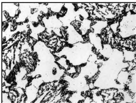
Балл 8, 500 х , химическое травление
