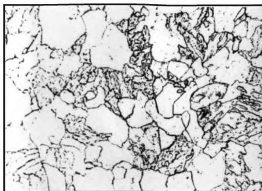
Балл 3, 500 х , химическое травление
