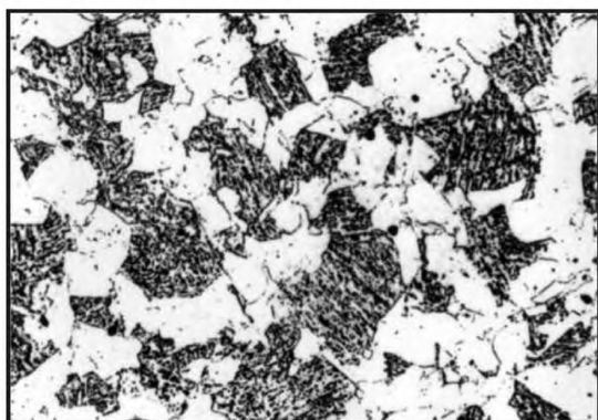
Балл 4, 100 ×
