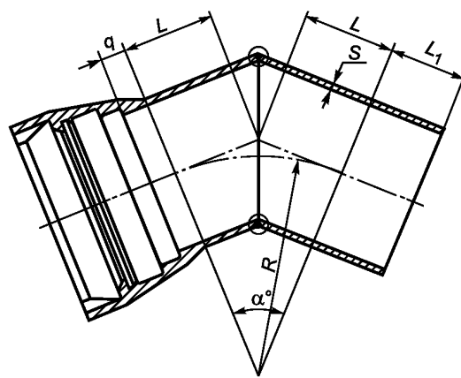
б) Отвод, раструб – гладкий конец (ОРГ)
