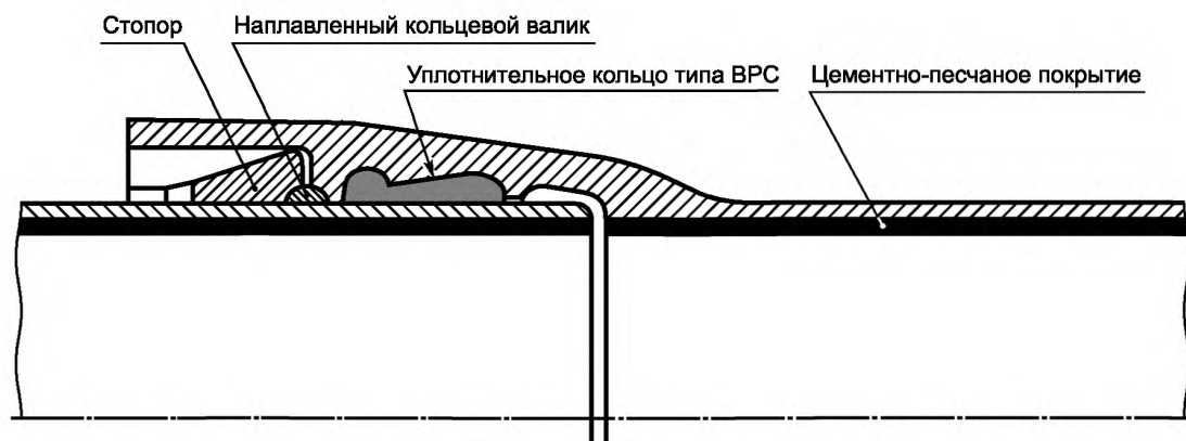
а) С уплотнительным резиновым кольцом типа «ВРС»
