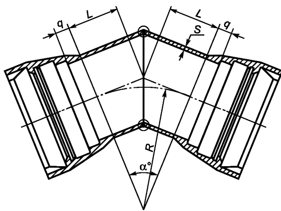
а) Отвод раструбный (ОР)
