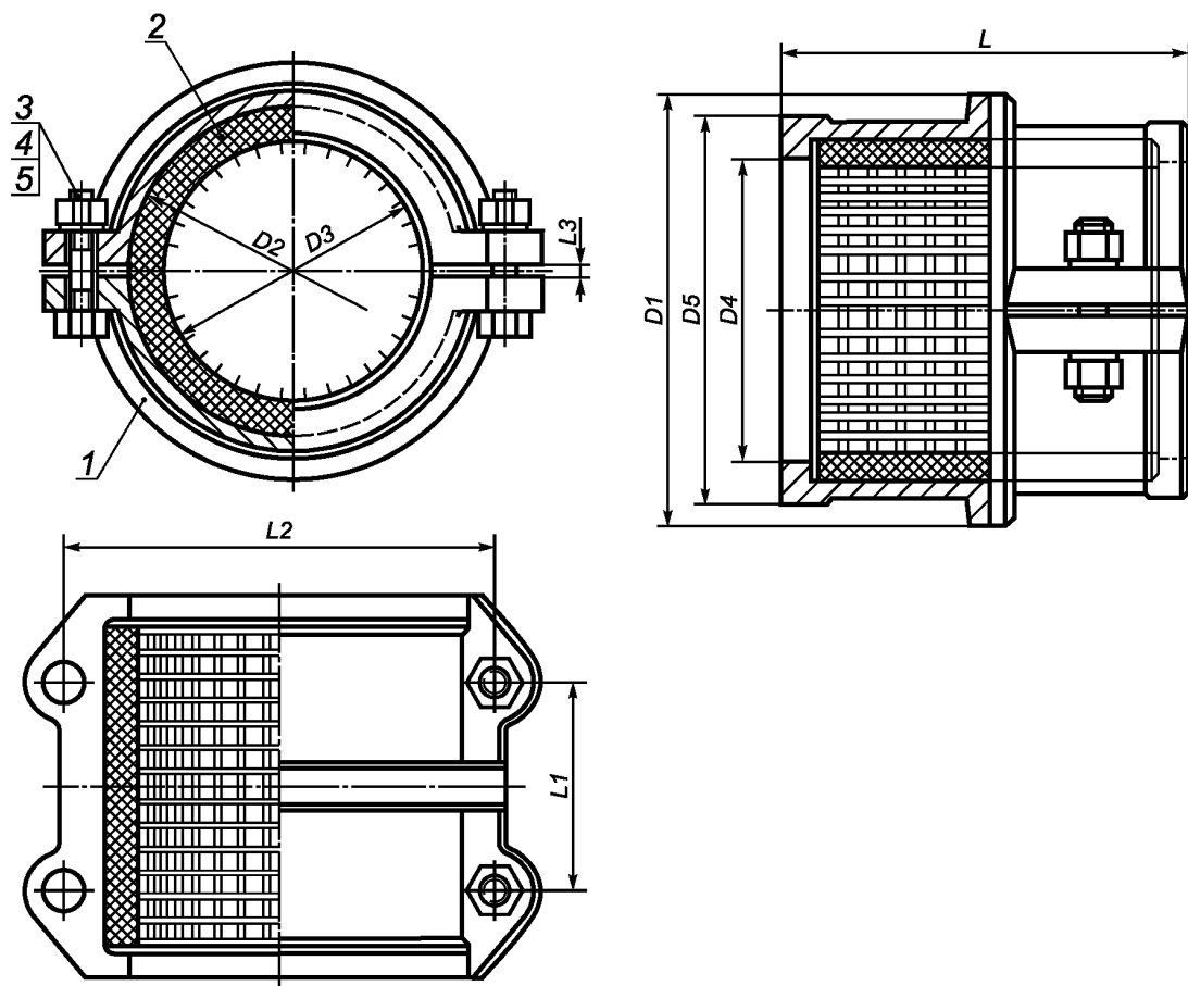
Рисунок Б.11 — Муфта свертная (МС)
