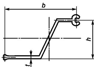
Рисунок 2 — Поперечное сечение зетовых композитных шпунтов
