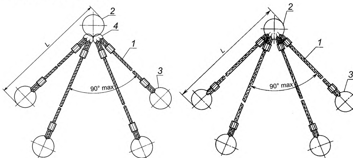
Рисунок 4 — Четырехветвевый канатный строп исполнения 1
