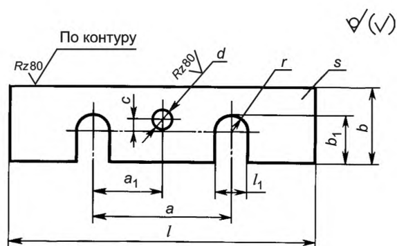
Рисунок Б.3 — Ограничитель Ог для звеньев Рт
