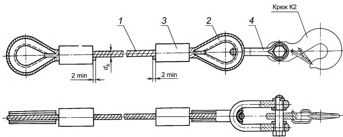
Рисунок А.1 — Канатная ветвь с заделкой концов каната опрессовкой алюминиевой или стальной втулкой (а) и с заделкой концов каната заплеткой (б)
