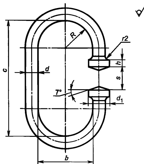
Рисунок Б.14 — Скоба Сов для звеньев Ров грузоподъемностью до 2,00 тс
