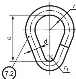
Рисунок Б.24 — Звено О
