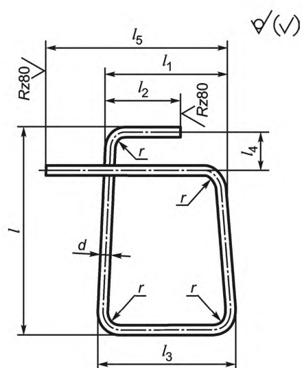
Рисунок Б.36 — Замок 32 для захвата К2
