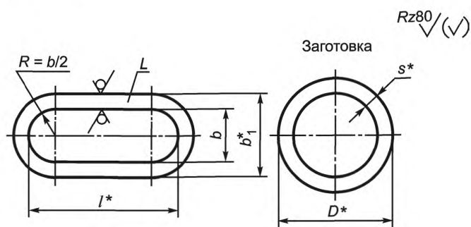
Рисунок В.3 — Стальная втулка СВт
