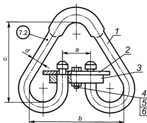
1 — скоба; 2 — ограничитель; 3 — планка; 4 — болт по ГОСТ 7798; 5 — гайка по ГОСТ 5919; 6 — шплинт по ГОСТ 397
