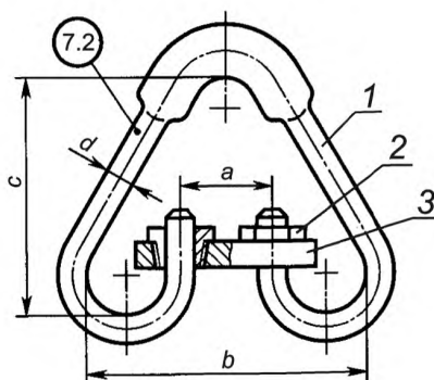
1 — скоба; 2 — гайка (2 шт.); 3 — планка
