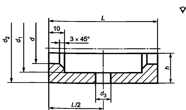
Рисунок Б.15 — Полумуфта Пм для звеньев Ров грузоподъемностью до 2,00 тс
