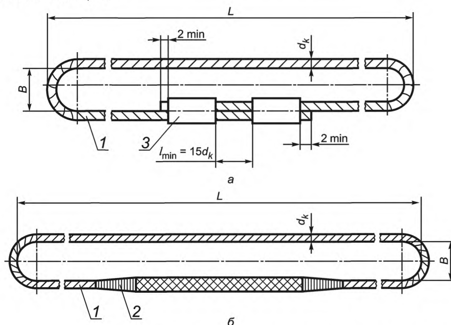
Рисунок 8 — Строп канатный кольцевой исполнения 1 с заделкой концов каната опрессовкой алюминиевой втулкой (а) и с заделкой концов каната заплеткой (б)
