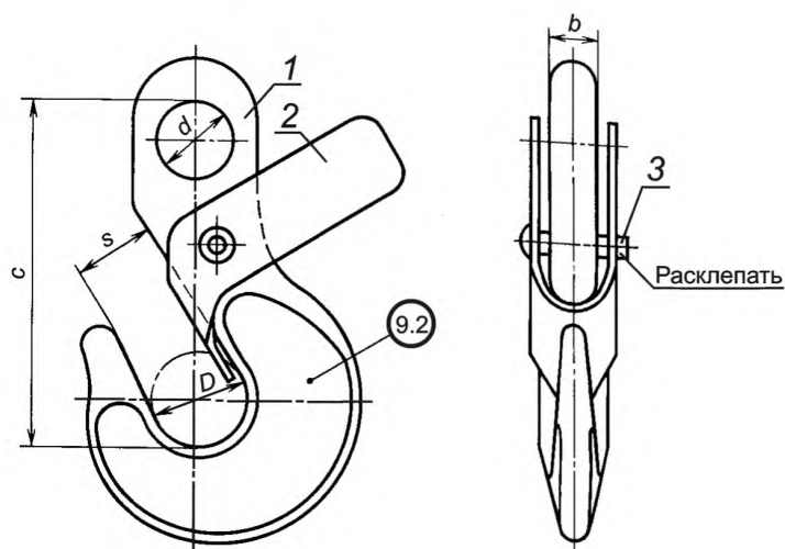
1 — крюк чалочный; 2 — замок; 3 — заклепка
