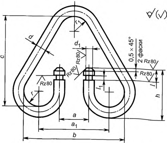
Рисунок Б.2 — Скоба Ст1 для звеньев Рт1
