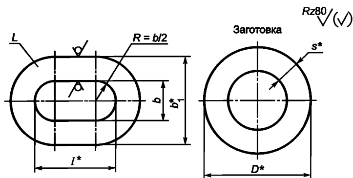
Рисунок В.2 — Алюминиевая втулка Вт
