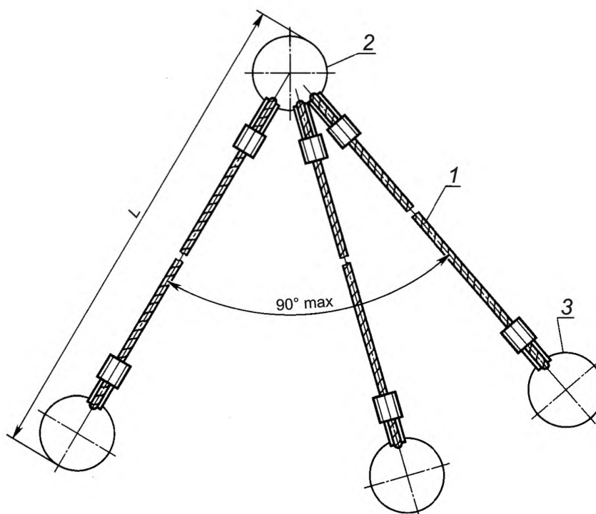
Рисунок 3 — Трехветвевой канатный строп
